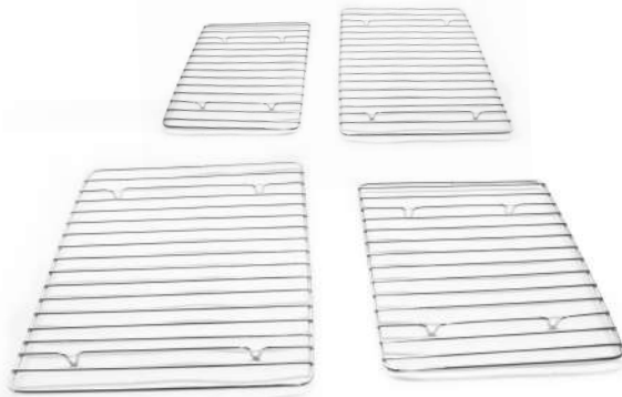
C. 1134- Rejilla para horno N°1 - 200x270 C. 1135- Rejilla para horno N°2 - 240x330 C. 1136- Rejilla para horno N°3 - 270x370 C. 1137- Rejilla para horno N°4 - 320x420
